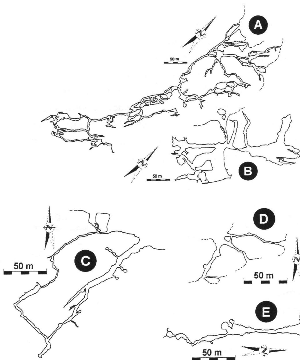
Figura 2: Cavernas do DI. (A) Gruta das Bromélias, 2750 m de desenvolvimento linear-DL; (B) Grutadas Casas, 600 m DL; (C) Gruta do Bocão 494 m DL; (D) Gruta dos Fugitivos, 186 m DL; (E) Gruta do Pião, 126 m DL. Ver texto para detalhes. Mapas simplificados; cortesia SPEC.
