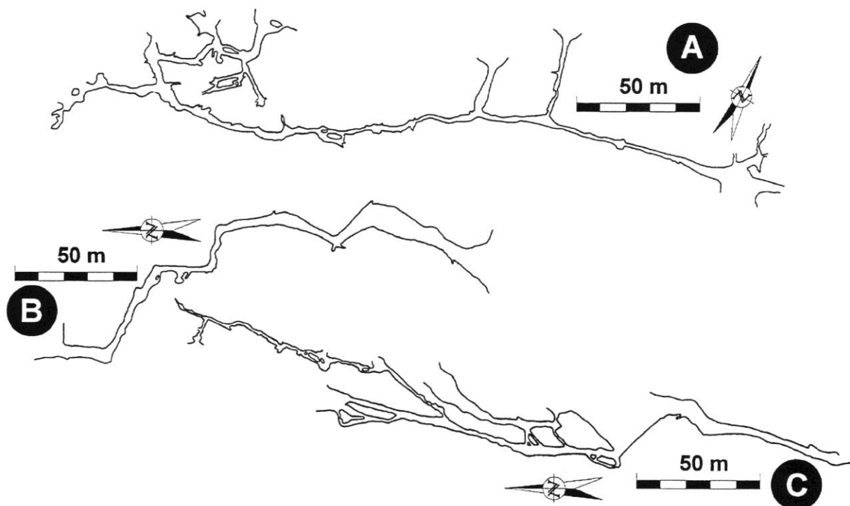
Figura 3: Mapas simplificados de cavernas dos DC (A) e DL (B) e (C). (A) Toca de Carrancas, 583 m DL; (B) Toca do Chico Lino, 213 m DL; (C) Tocas Num Sei I e II, 408 m e 60 m DL; (B) e (C) cortesia GBPE. Ver texto para detalhes.
