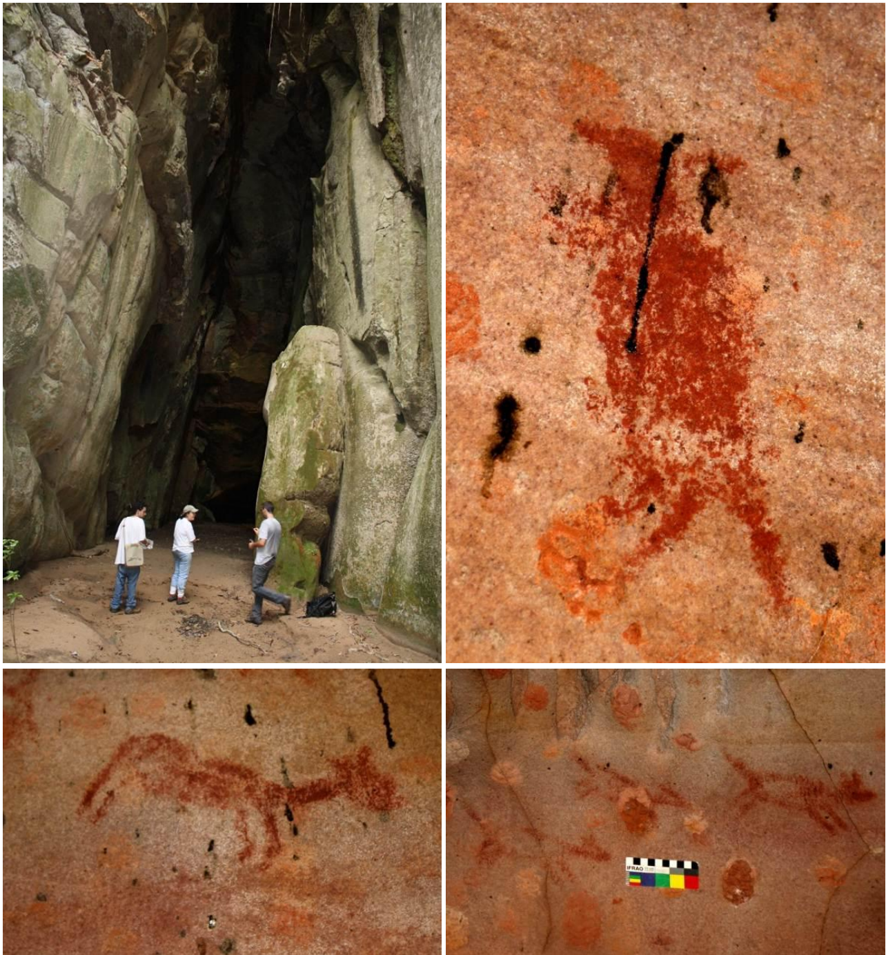
Figura 6: A Caverna Grande do Taboco e suas pinturas
