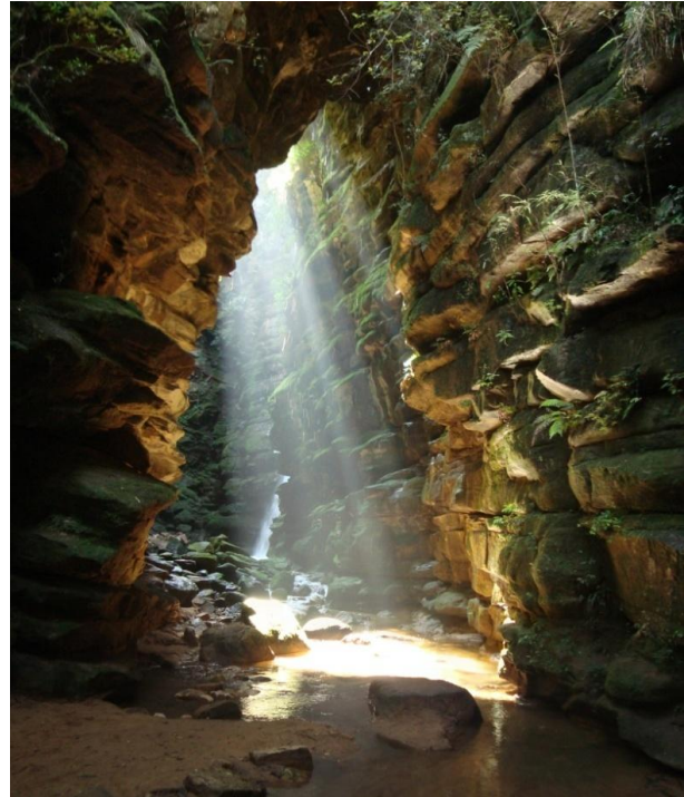
Figura 02: Buraco do Padre - Ponta Grossa-PR, acesso principal por rio subterrâneo
