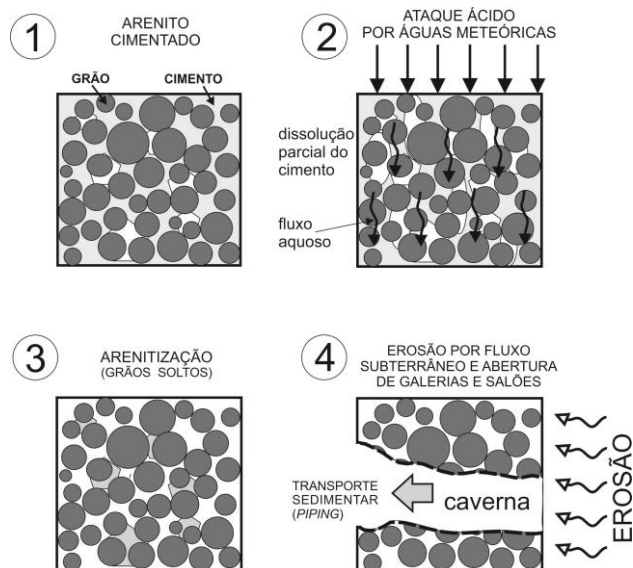
Figura 09- Esquema para explicar o processo de dissolução do cimento de arenitos por ação de águas meteóricas, conduzindo a rocha à fragilidade ( arenitização ) mecânica e favorecendo a ação de erosão por fluxo hidráulico ( piping ). Esse caminho dá início à formação da caverna em condições freáticas (veja texto para mais detalhes).
