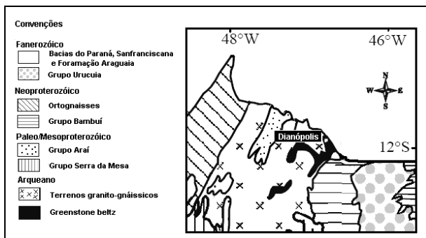
Figura 2 – Mapa geológico da região de Dianópolis e entorno (adaptado de DÁVILA; KUYUMJAM, 2005).
