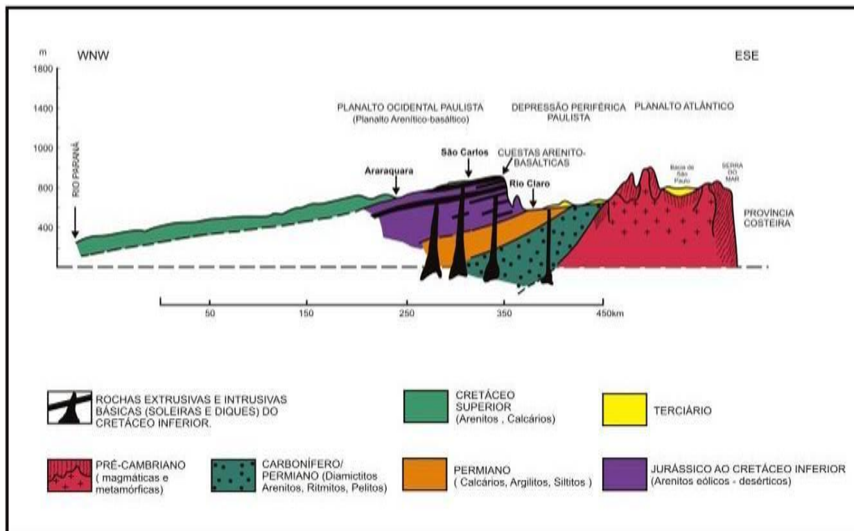
Figura 2 – Perfil geomorfológico do Estado de São Paulo (Modificado de Ab´Saber, 1956).
