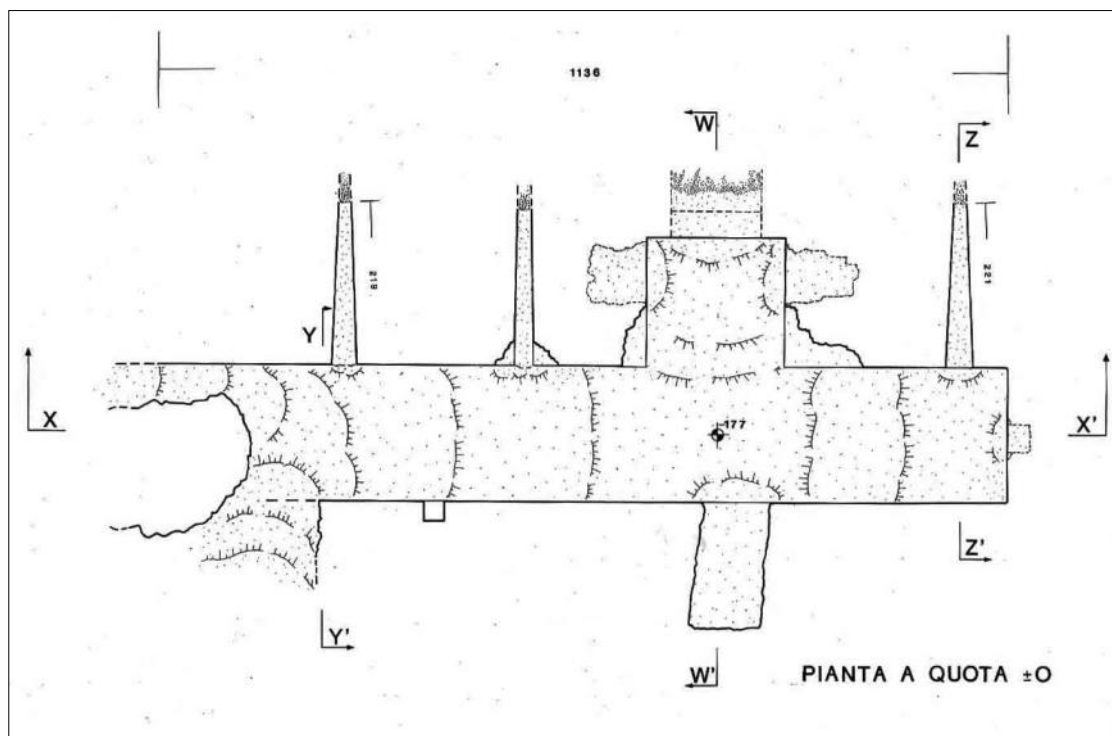
Fig. 18 - Pianta di un tratto della Galleria di Controscarpa del Bastione di Sant'Ignazio (CA 00001 PI CN).
