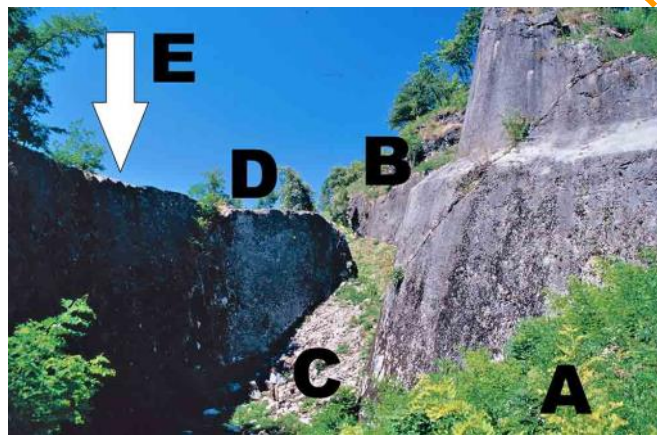
Fig. 15c - In dettaglio: A- "Tenaglione verso Stura", B- scarpa della cortina tagliata nella viva roccia, C- fossato (probabilmente si tratta di "fosso diamante"), D- controscarpa tagliata nella roccia, E- opere esterne alla controscarpa (spalto, galleria di controscarpa con feritoie, sortite, contromine, opere di deflusso delle acque dal fossato).
