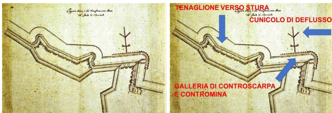
Figg. 40 e 40a. Il Tenaglione verso Stura, il Bastione di Sant'Ignazio, la Galleria di Controscarpa, il Cunicolo di Contromina e il Cunicolo di Deflusso dalla cui camera circolare si staccano i tre condotti per l'esfiltrazione dell'acqua (Viglino Davico M., Fortezze sulle Alpi. Difese dei Savoia nella Valle Stura di Demonte , Edizioni L'Arciere, Cuneo 1989, p. 192, tav. D 33 a [ISCAG, FO Demonte]). Analogo impianto difensivo di controscarpa con contromine e opere di deflusso dovrebbe proteggere il fianchi salienti del Bastione Sud dell'Opera a Corno.
