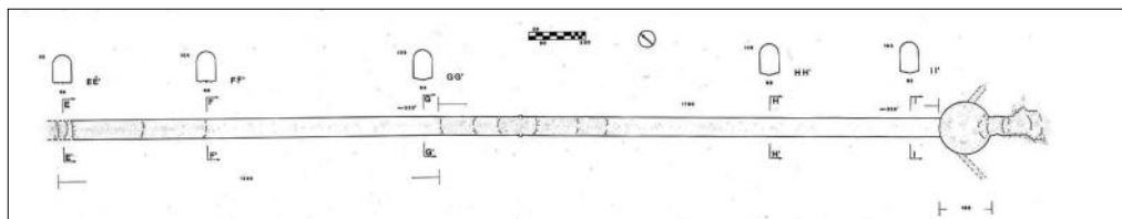
Fig. 39 - Pianta del Cunicolo di Deflusso del Bastione di Sant'Ignazio (CA 00003 PI CN).
