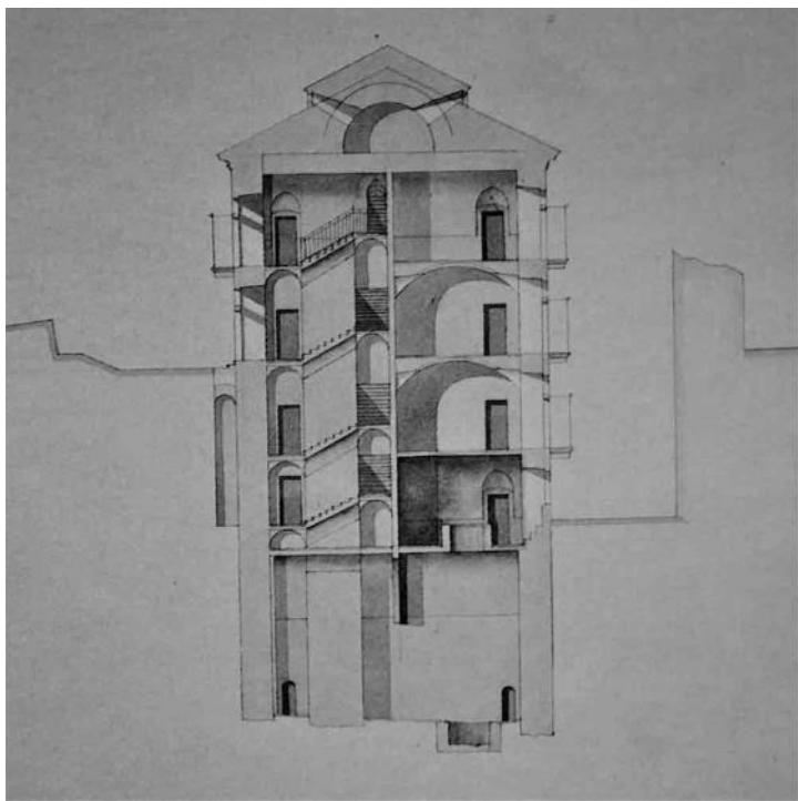
Fig. 75 - Forte di Demonte: edificio “alla prova” con più livelli sotterranei scavati nella viva roccia (Esercito Italiano, Istituto Storico e di Cultura Arma del Genio, Forte Demonte).
