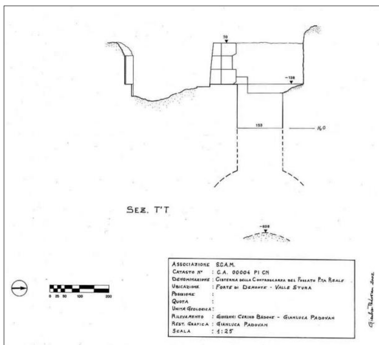
Fig. 48 - Cisterna della Controscarpa del Fossato della Porta Principale (CA 00005 PI CN): sezione.
