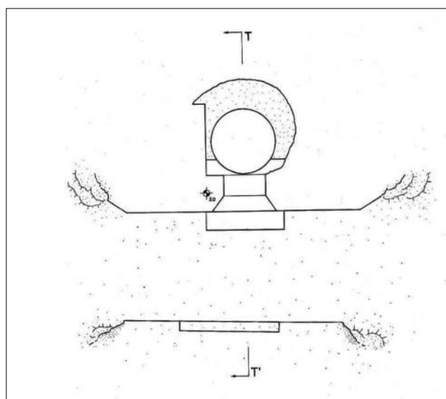
Fig. 49. Cisterna della Controscarpa del Fossato della Porta Principale (CA 00005 PI CN): pianta.
