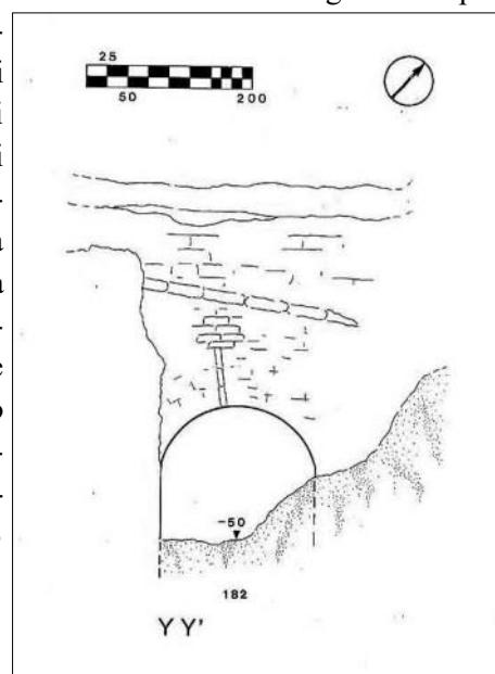
Fig. 19 - Sezione trasversale della Galleria di Controscarpa del Bastione di Sant'Ignazio (CA 00001 PI CN).
