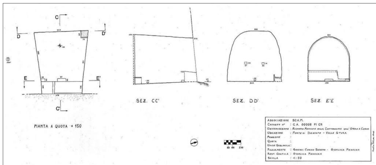
Fig. 52 - Ricovero Maggiore nella Contrascarpa dell'Opera a Corno (CA 00005 PI CN).
