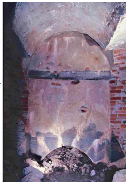
Fig. 27 - Accesso alla Posterla, integro ma interrato.
