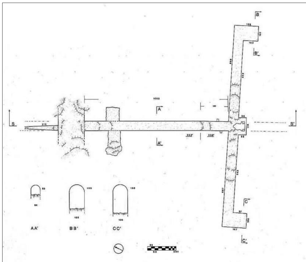
Fig. 30 - Pianta dell'impianto di Contromina (CA 00002 PI CN).
