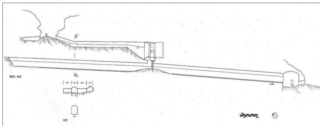
Fig. 29. Sezione dell'impianto di Contromina (CA 00002 PI CN) con sottostante Cunicolo di Deflusso (CA 00002 PI CN).
