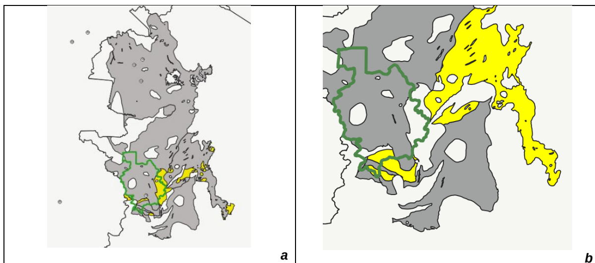
Figura 69 - a) Áreas da Suíte Ataléia (em amarelo escuro) excluídas (baixo ou médio potencial) das áreas prioritárias para prospecção espeleológica Espirito Santo (em cinza); b) Áreas da Suíte Ataléia (em amarelo) mantidas (alto ou muito alto potencial). Em verde, limite do município de Pancas.
